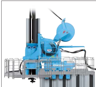
作业平台
