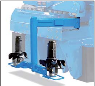
钻头更换装置
