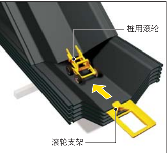
桩用滚轮
